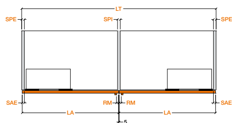
●俯視剖面圖2
